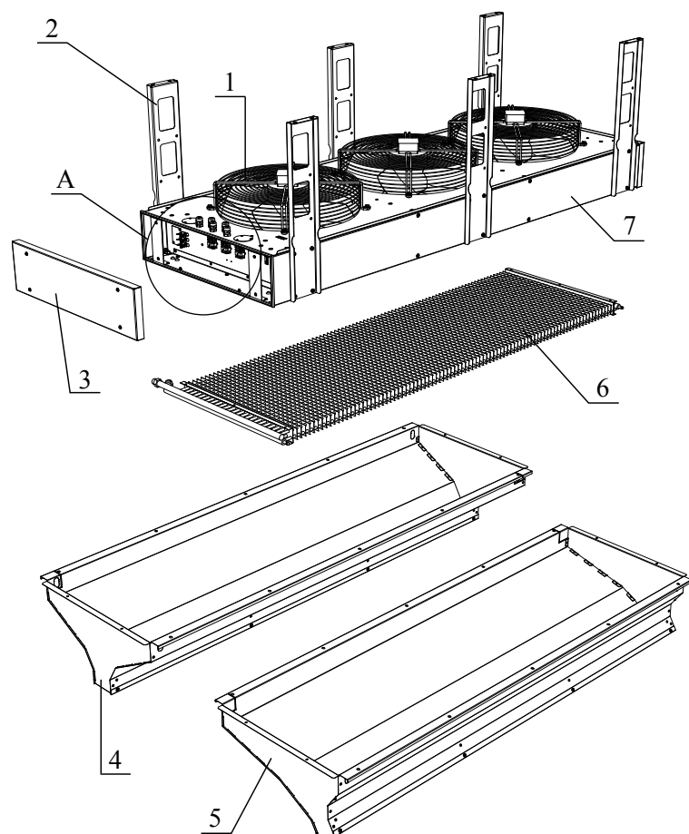
Рисунок 2. Воздушно-тепловая завеса
